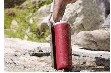
3 Sicherheit: Die Cracker werden mit Hilfe eines Patronenhalters in das Loch eingefügt. Event. Blindgänger könne so auch wieder aus dem Loch entfernt werden.
